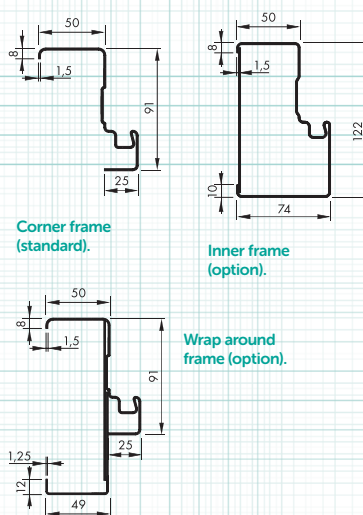
Fig. 2 Frame options
